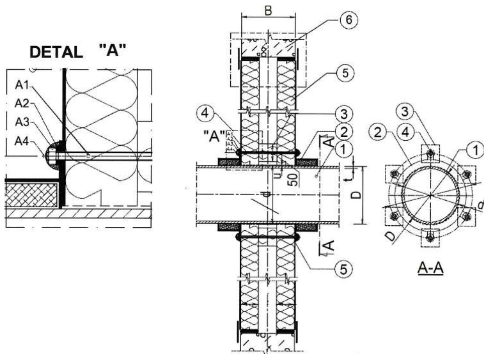
Rys. C28. Uszczelnienie mieszanego przejścia rury z tworzywa sztucznego ścianą sztywną, wykonane za pomocą Flame Cabel Pasta A i CarboCollar CC
