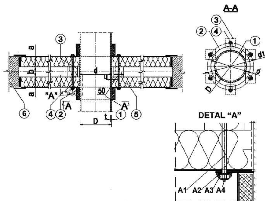
Rys. C29. Uszczelnienie mieszanego przejścia rury z tworzywa sztucznego przez strop sztywny, wykonane za pomocą Flame Cabel Pasta A i CarboCollar CC
